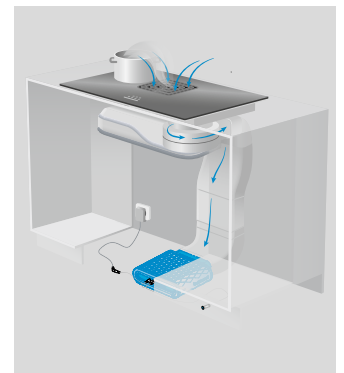
Circuit fermé avec filtre plasma
