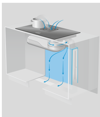
Circuit fermé avec filtre Permalyt®
