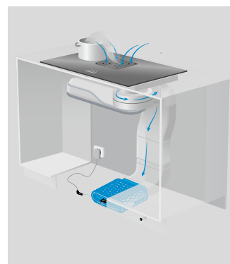
Circuit fermé avec filtre plasma
